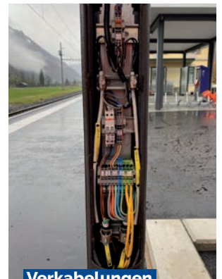
Verkabelungen Kombiständer
