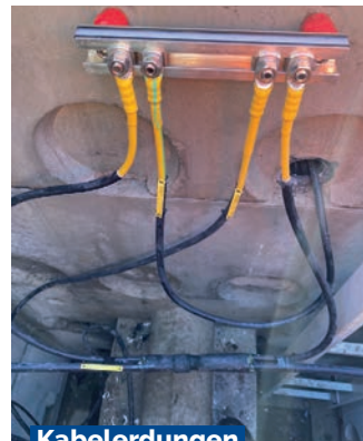
Kabelerdungen in Kabelschacht
